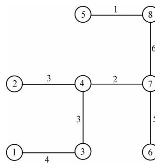
图 3 光纤铺设方案
