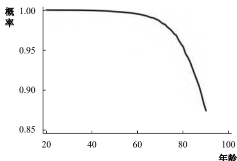
图 2 条件生存概率
